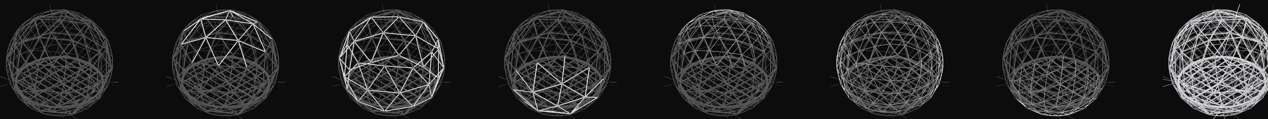
secuencia de perspectivas isométricas de los diferentes grupos de barras según su criterio de dimensionado que componen la estructura de la cúpula geodésica
