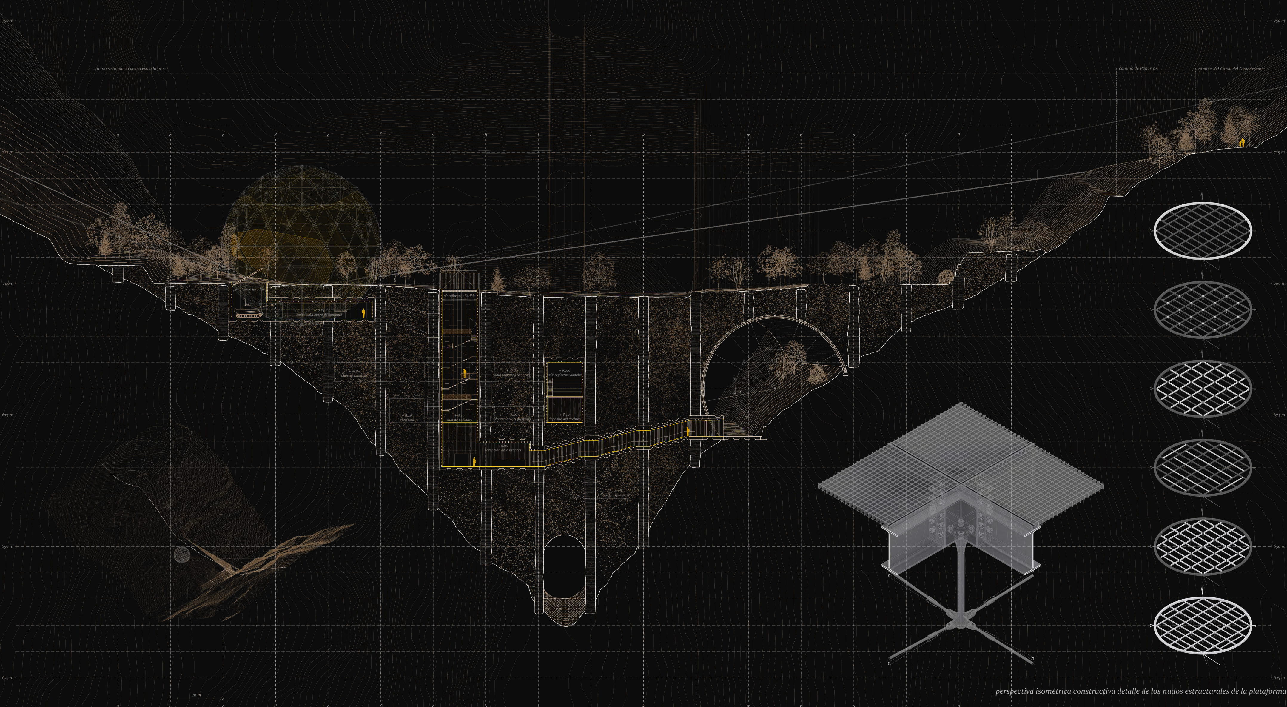
sección longitudinal sur de la presa de El Gasco tomada desde su vista aguas abajo con plano topográfico superpuesto
