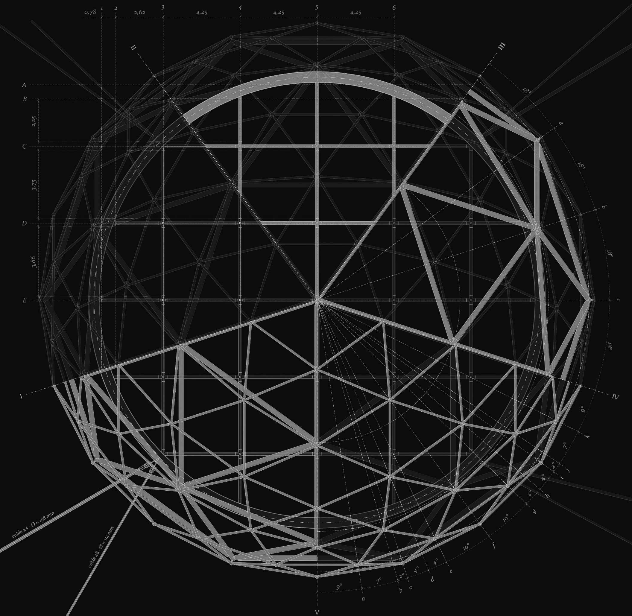
secuencia de alzados detalle de las costillas transversales que componen la estructura de la sala de conferencias
